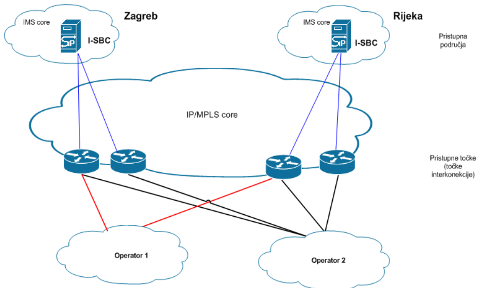
Slika 1. Arhitektura SIP međupovezivanja s HT mrežom
